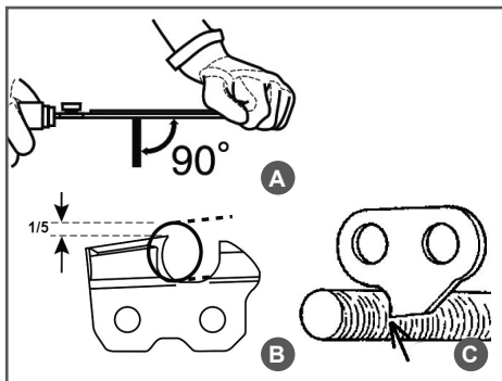
Рис. 17 Заточка цепи
